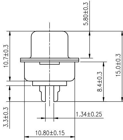
端子图 SCALE:2.1
