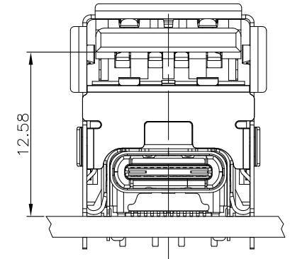
HIGE RISE USB2.0+USB TYPE-C
